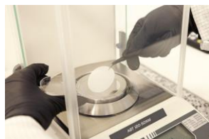
Gravimetrie
